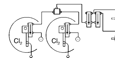
Modelo Hydro 702-2 Reserva Automática con Múltiples Puntos de Alimentación
